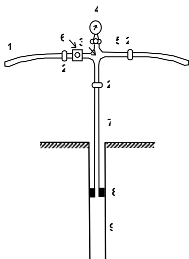
Gambar B.1 Rangkaian peralatan injeksi dan bagian-bagiannya
