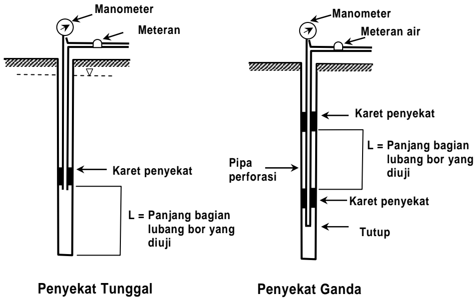
Gambar B.3 Cara pemasangan karet penyekat
