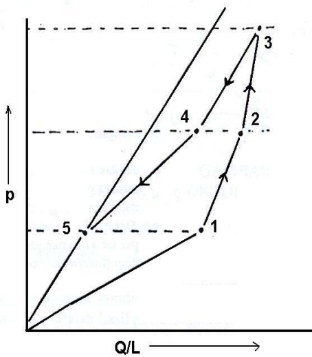
Gambar B.10 Grafik aliran p-Q/L untuk penyumbatan
