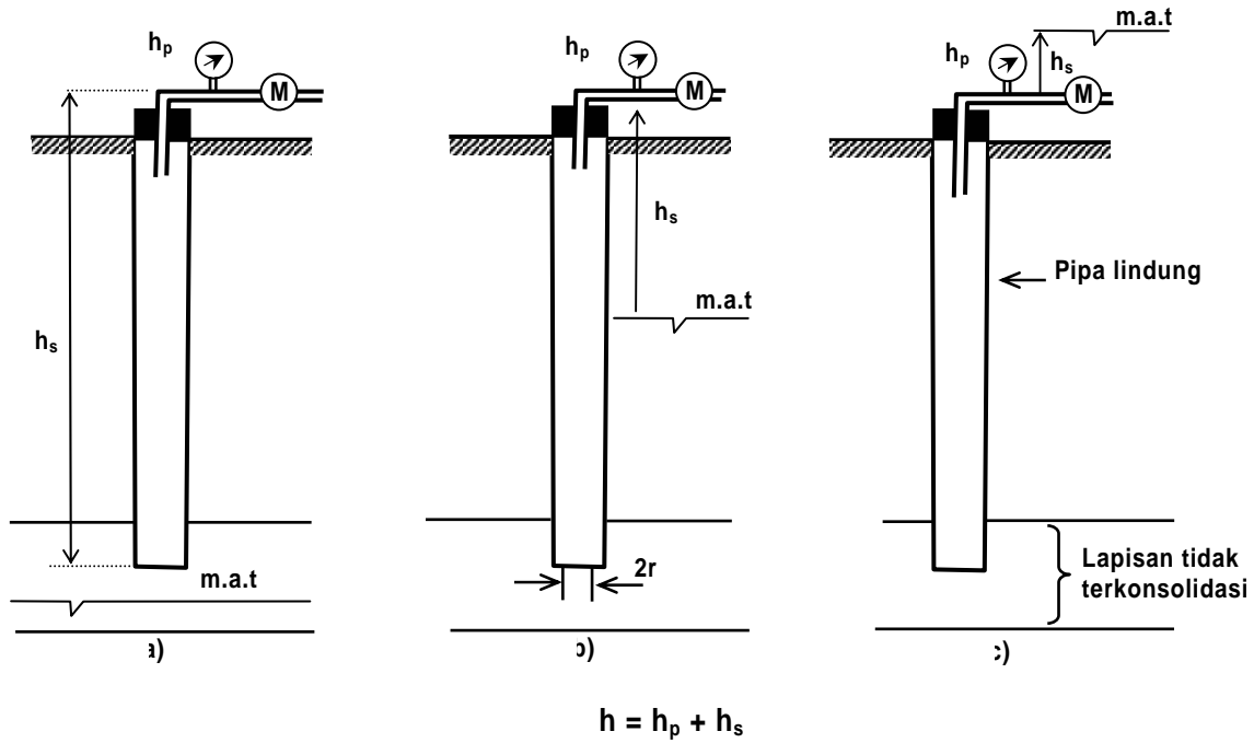
Gambar B.11 Pelaksanaan uji kelulusan air bertekanan pada bagian tanah yang bersifat tidak terkonsolidasi/lubang bor runtuh
