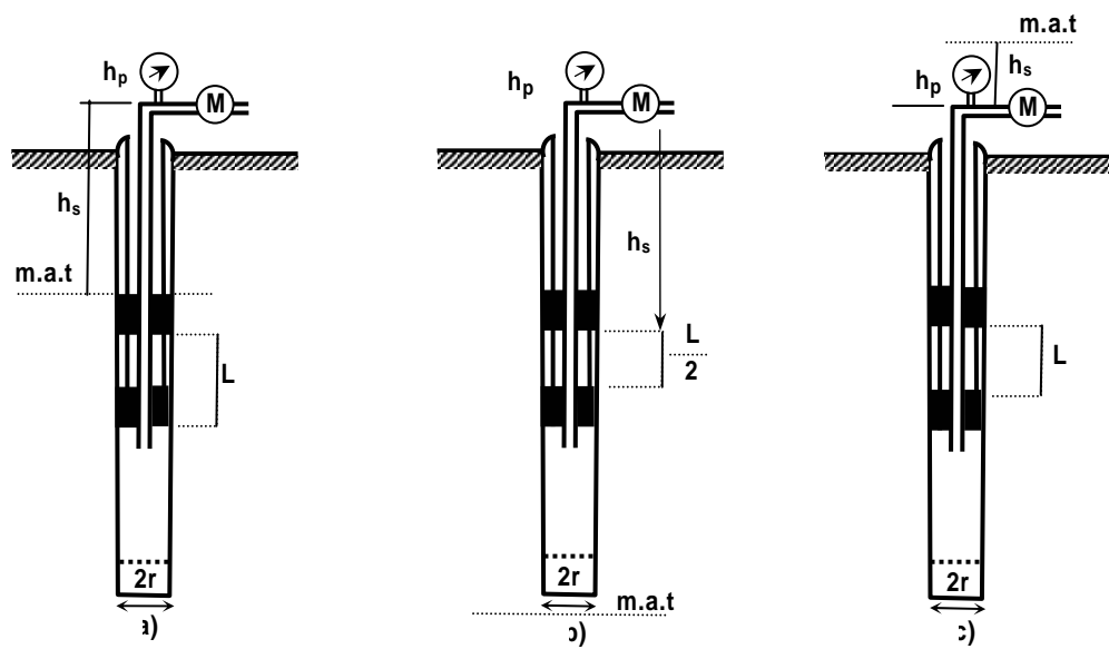
Metode Penyekat Ganda
