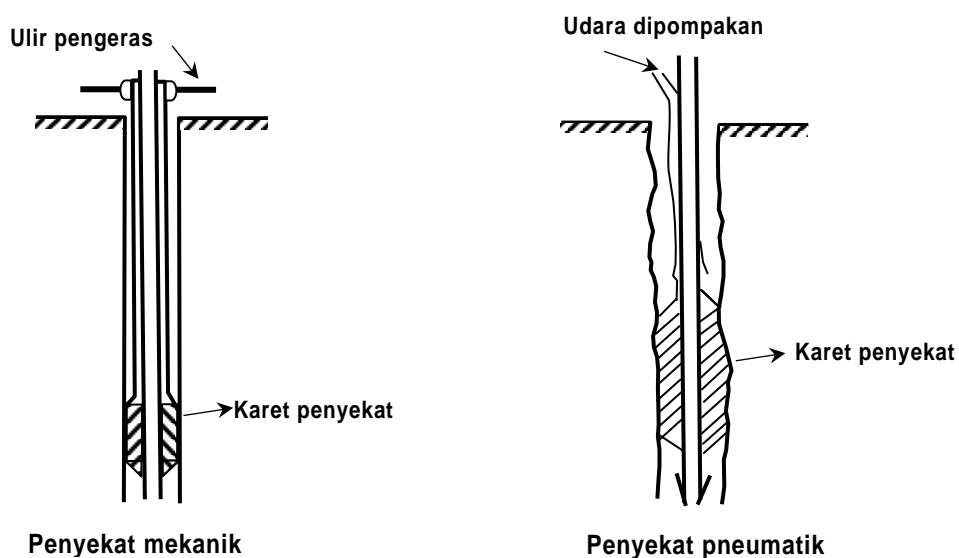
Gambar B.2 Jenis penyekat mekanik dan pneumatik
