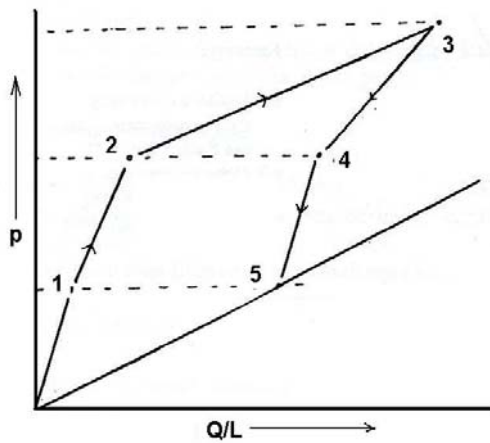
Gambar B.9 Grafik aliran p-Q/L untuk pengikisan
