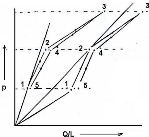
Gambar B.8 Grafik aliran p-Q/L untuk dilasi
