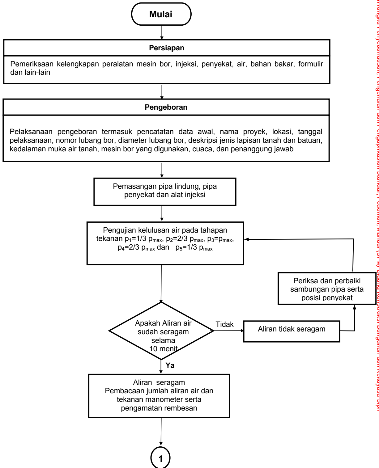
Gambar A.1 Bagan alir cara uji kelulusan air bertekanan di lapangan
