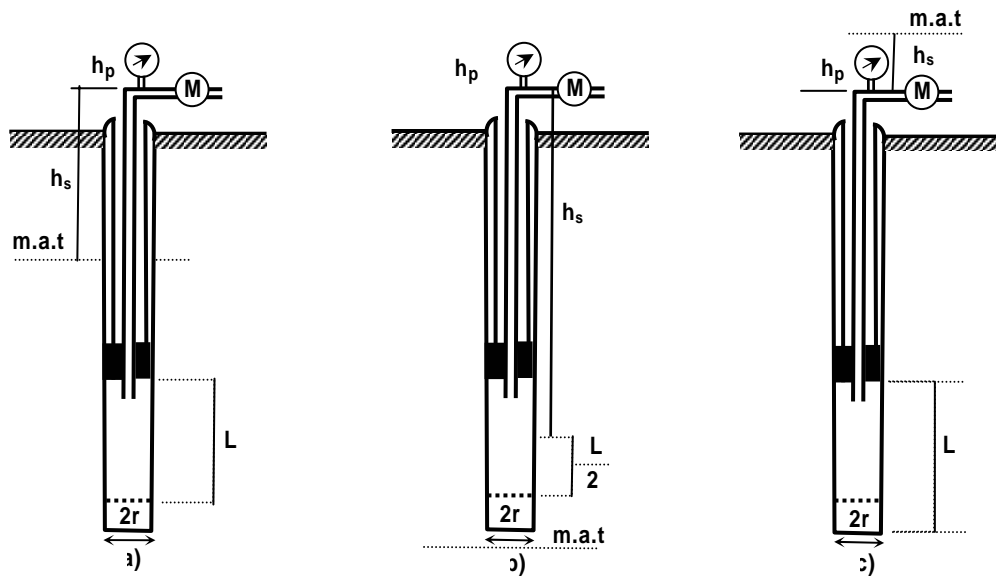
Metode Penyekat Tunggal
